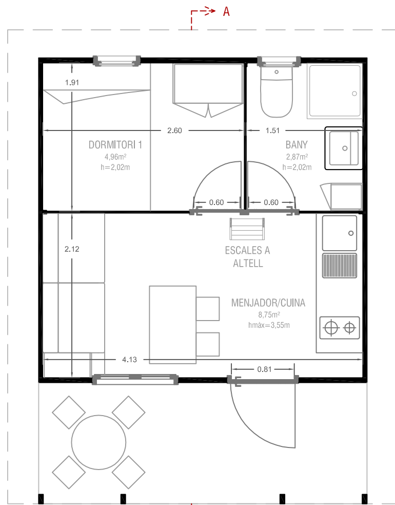
PLANTA BAIXA
